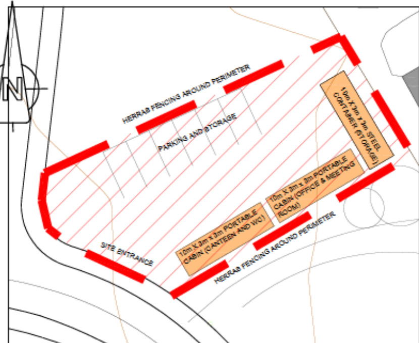
SITE PLAN 1:200
